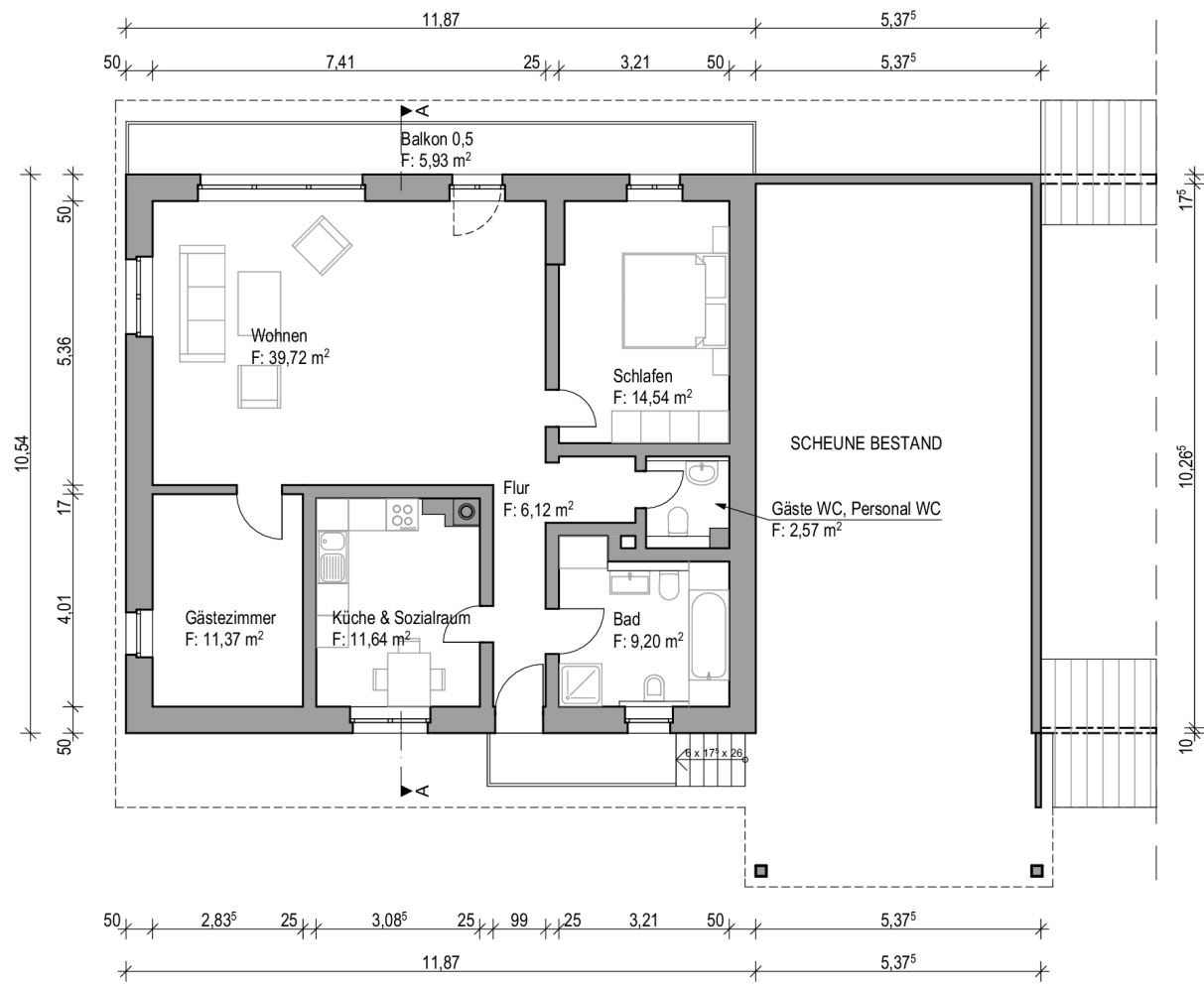
GRUNDRISS OBERGESCHOSS
